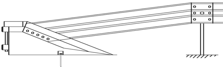
Prehodni element. Potrebno je sidranje v podlago.
